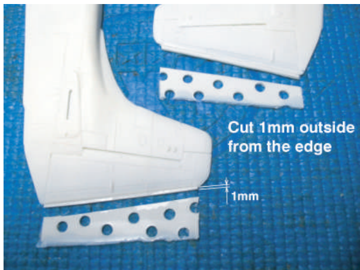
前処理 -1 Parts pretreatment -1
