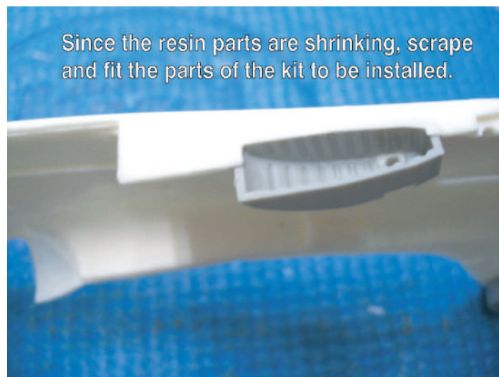
ベースキットとの嵌合 Matches of the base kit parts
