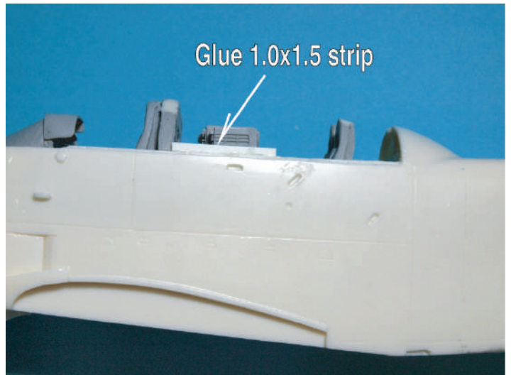
後部キャノピーの加工 -2 (重要) Rear canopy modification-2 (Important!)
